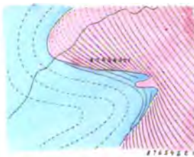
Fig. 2. Erste Hypothese zur Erklärung des Mettenbergs.
